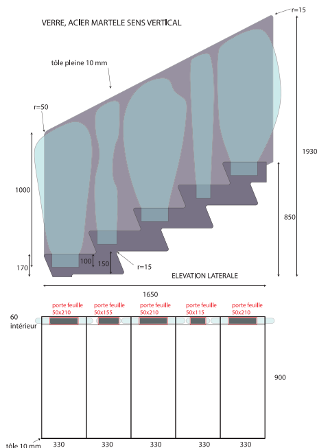
PROJET DE RAMPE D'ESCALIER
